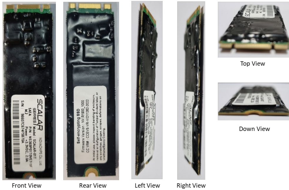
Figure 7. M.2 SATA 2280 SSD Module (NS369P01T0VE7-1F)
