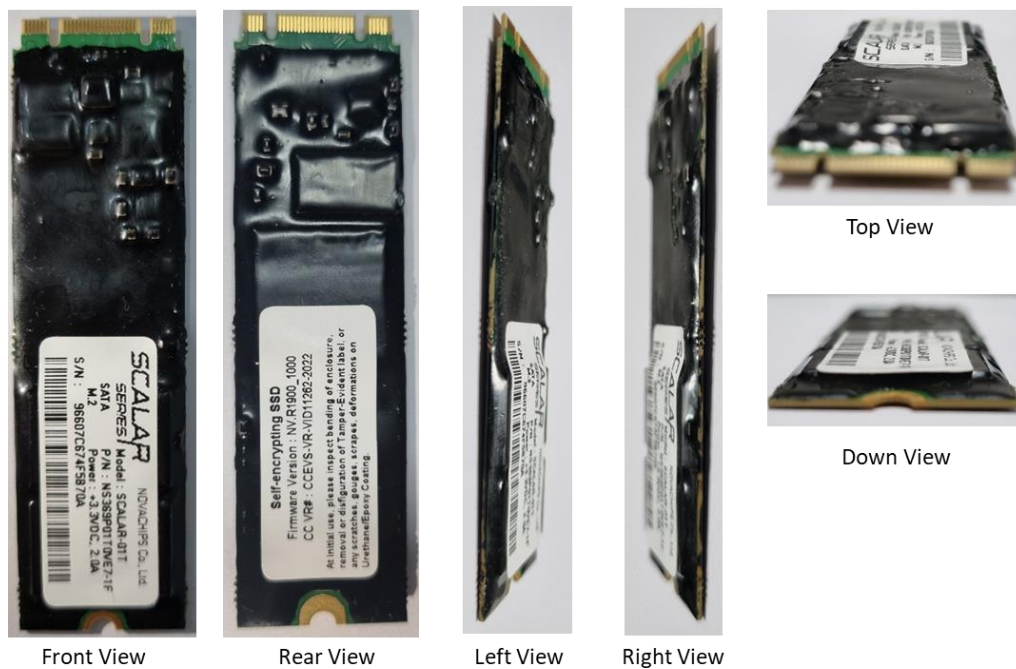
Figure 10. M.2 SATA 2280 SSD Module (NS369P01TOVE7-1F)
